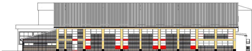
Projektowana hala sportowa, elewacja północno - wschodnia, skala 1:200
